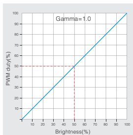
Linioowa krzywa ściemniania
